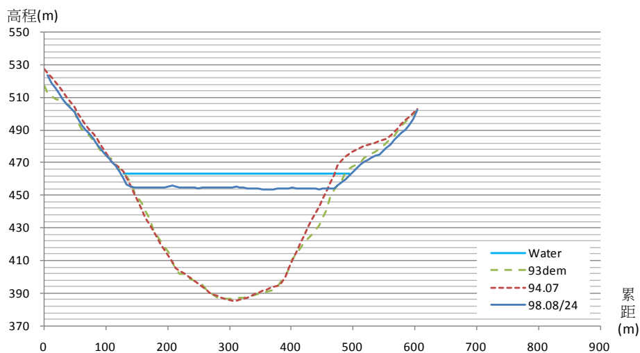
水下地形測量成果斷面 A5
