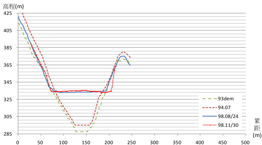
太麻里溪河道斷面比對断面 17
