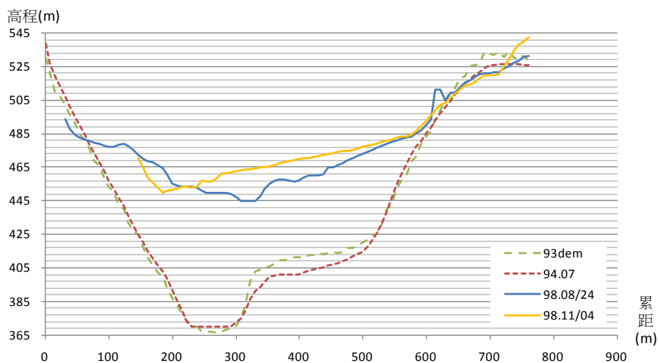
太麻里溪河道斷面比對斷面 23
