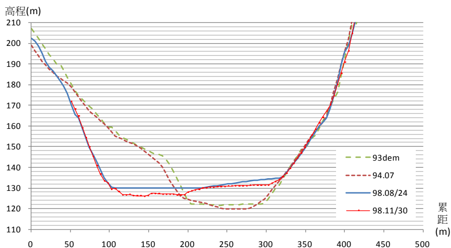
太麻里溪河道斷面比對断面 10
