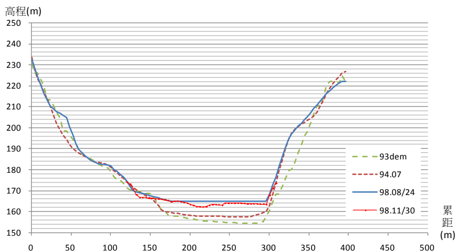
太麻里溪河道斷面比對断面 11
