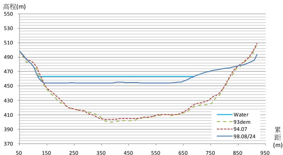
水下地形測量成果斷面 A9
