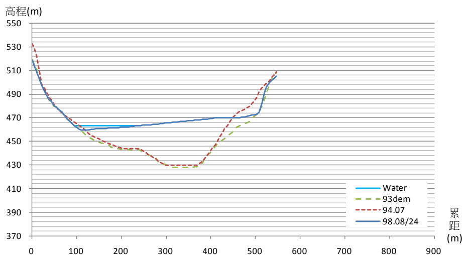
水下地形測量成果斷面 A13
