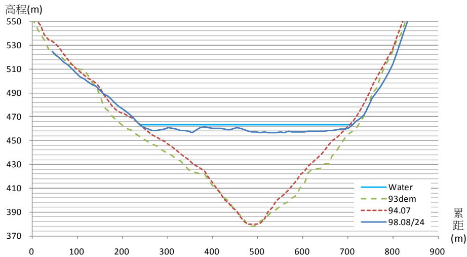
水下地形測量成果斷面 A2
