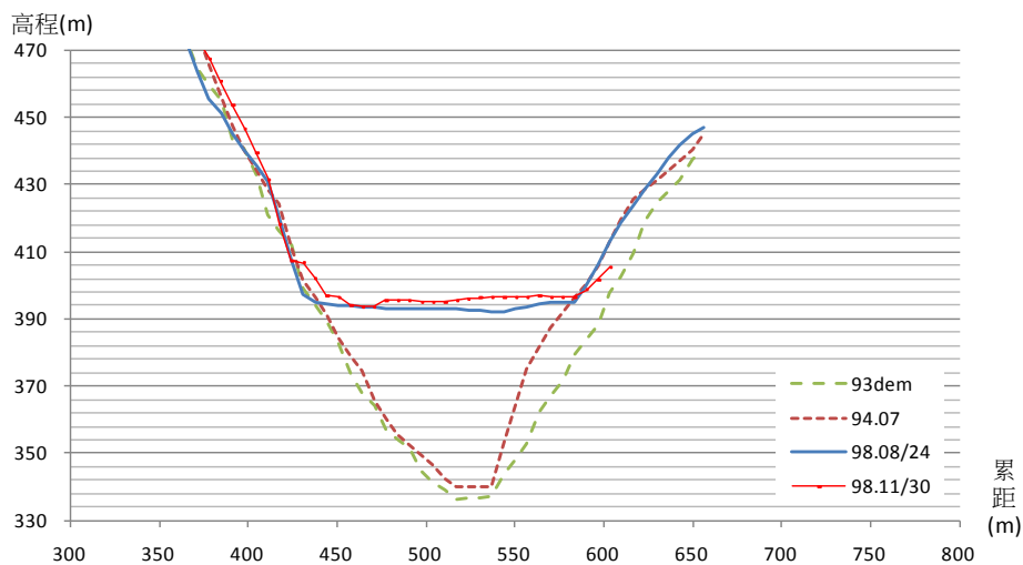
太麻里溪河道斷面比對斷面 21
