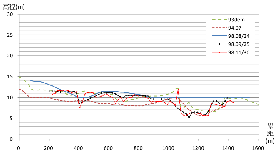
太麻里溪河道斷面比對斷面 1
