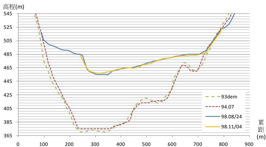
太麻里溪河道斷面比對斷面 24
