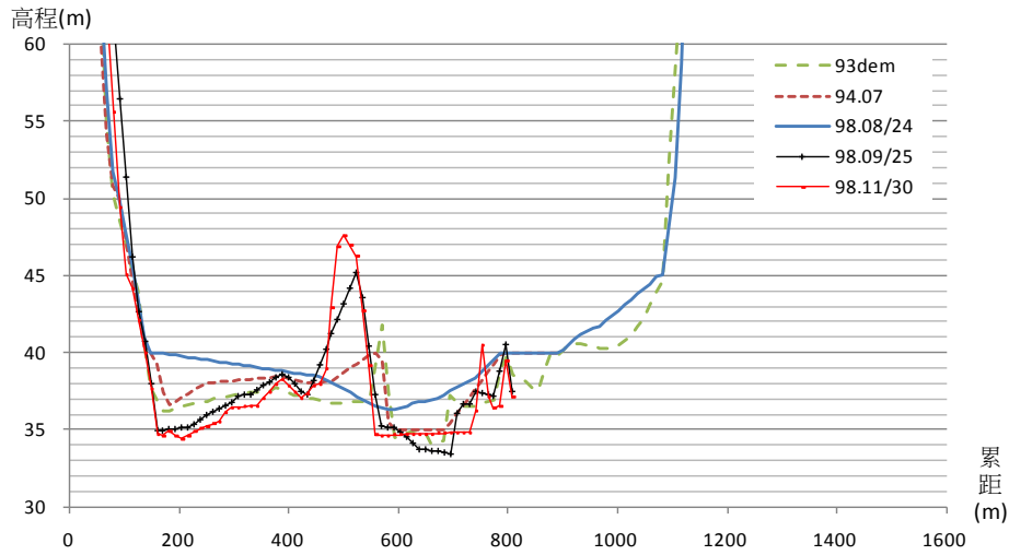
太麻里溪河道斷面比對斷面 3
