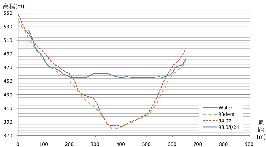
水下地形測量成果斷面 A3
