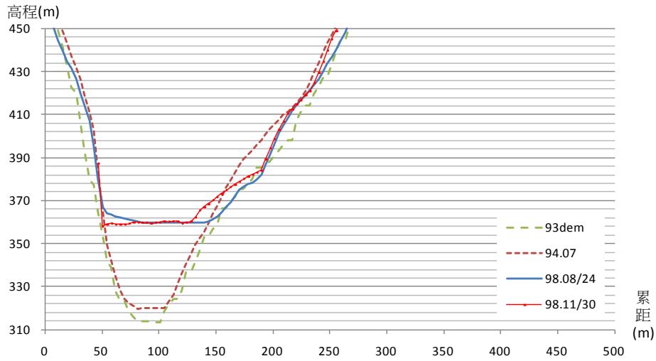
太麻里溪河道斷面比對断面 18
