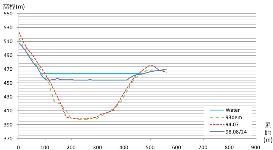
水下地形測量成果斷面 A8
