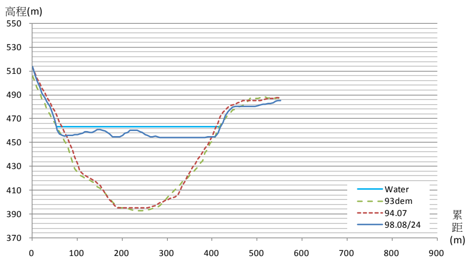
水下地形測量成果斷面 A7
