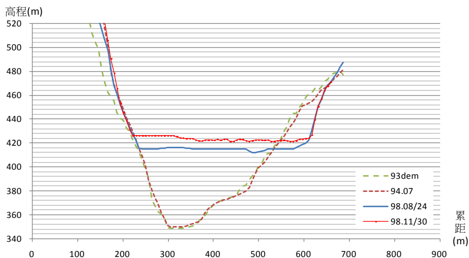
太麻里溪河道斷面比對斷面 22
