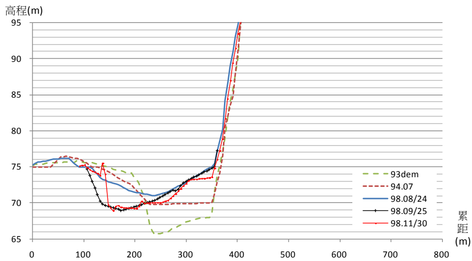
太麻里溪河道斷面比對斷面 7
