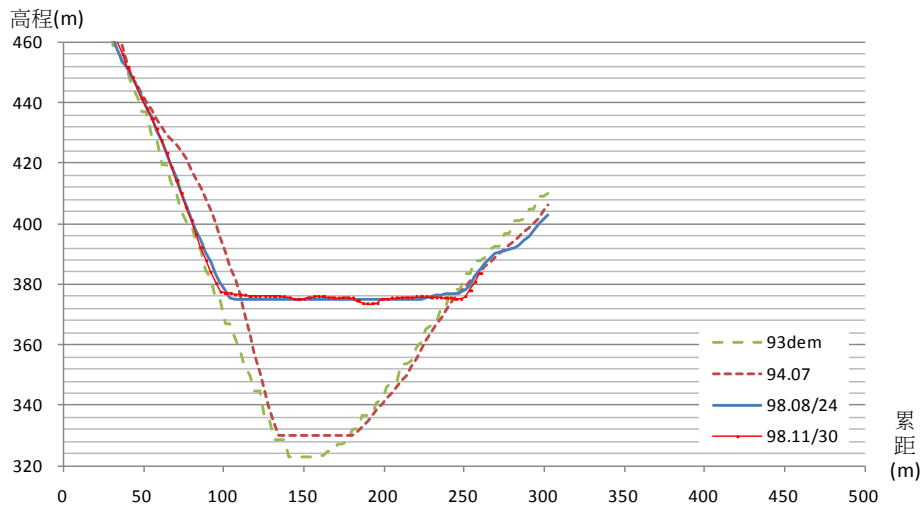
太麻里溪河道斷面比對断面 19
