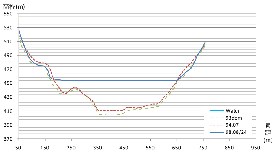
水下地形測量成果斷面 A10
