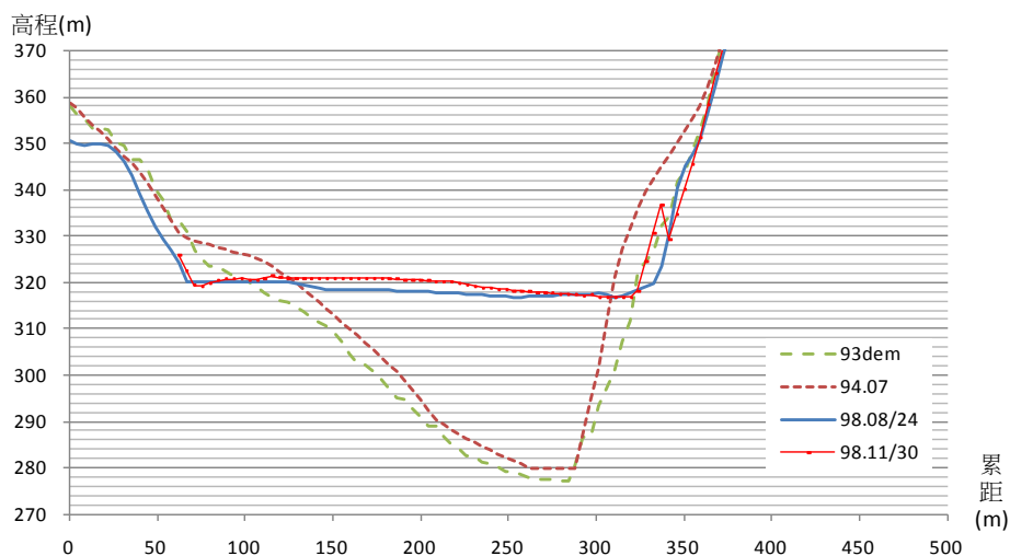
太麻里溪河道斷面比對断面 16
