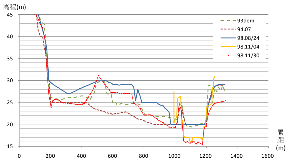
太麻里溪河道斷面比對斷面 2
