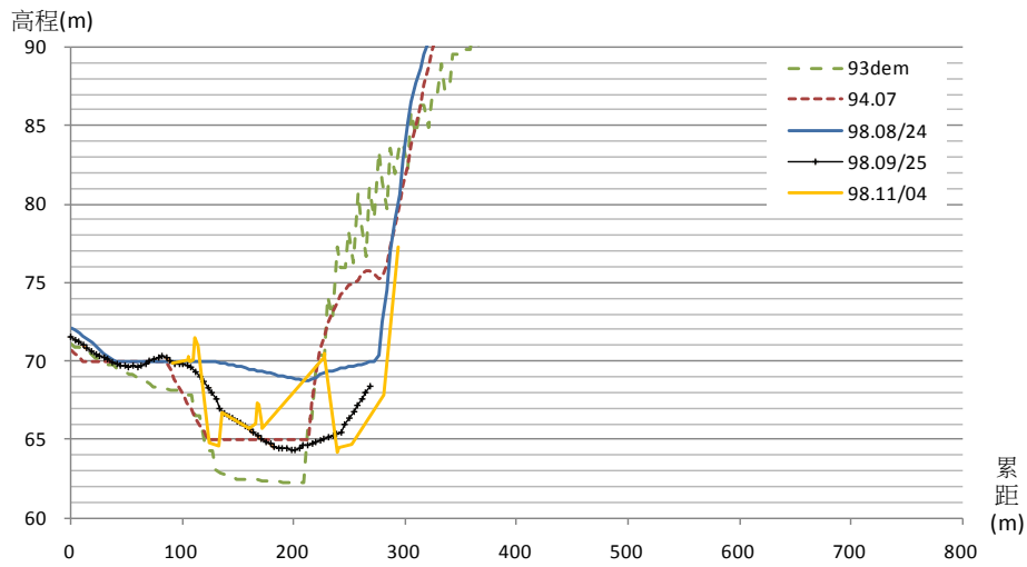
太麻里溪河道斷面比對斷面 6
