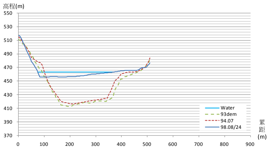
水下地形測量成果斷面 A12
