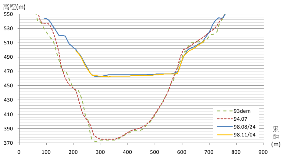
太麻里溪河道斷面比對斷面 25
