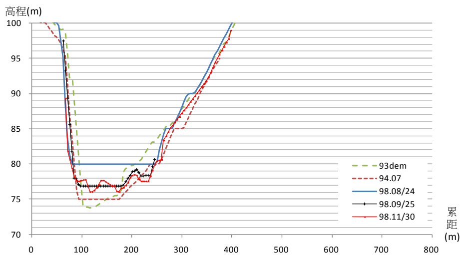
太麻里溪河道斷面比對斷面 8
