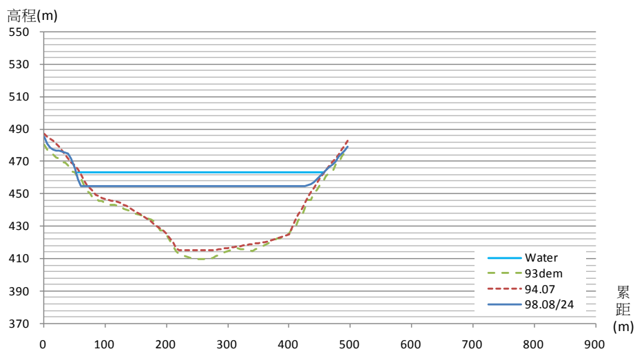
水下地形測量成果斷面 A11
