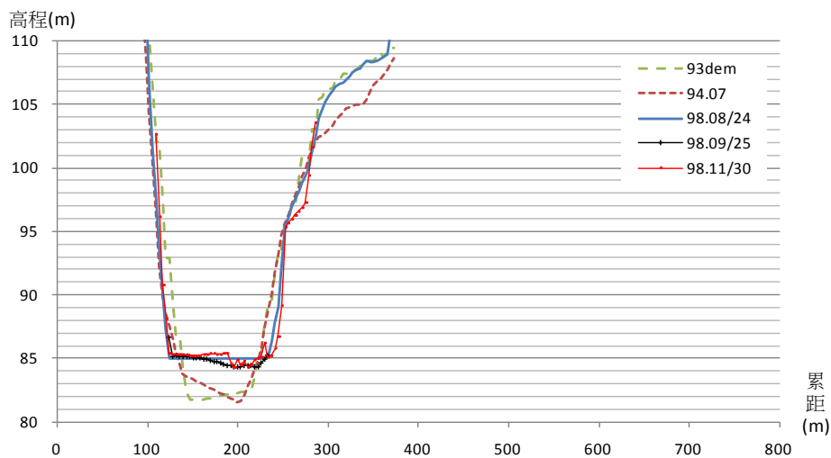
太麻里溪河道斷面比對断面 9
