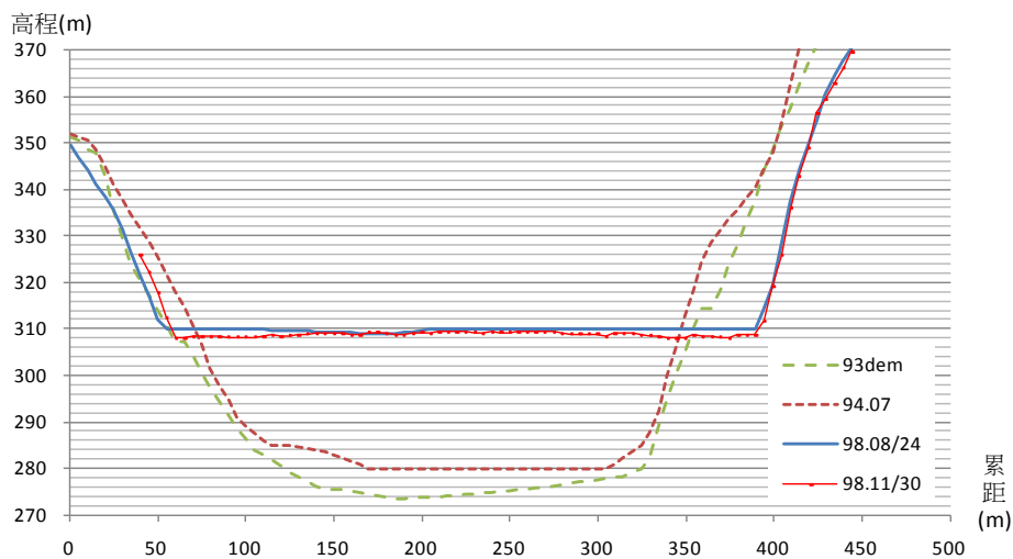
太麻里溪河道斷面比對断面 15
