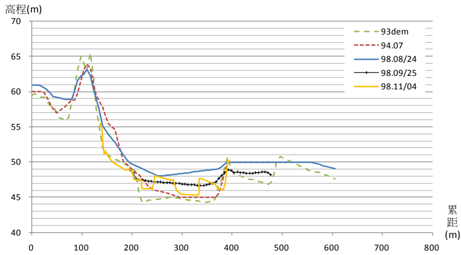
太麻里溪河道斷面比對斷面 4
