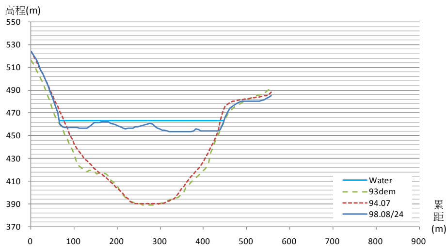
水下地形測量成果斷面 A6
