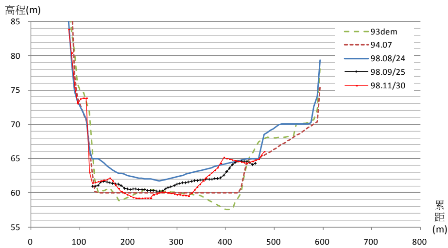
太麻里溪河道斷面比對斷面 5
