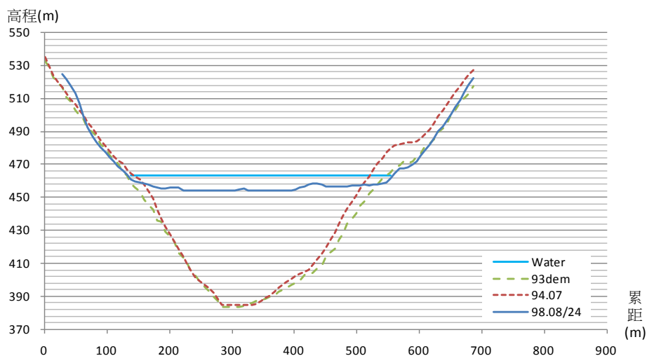
水下地形測量成果斷面 A4
