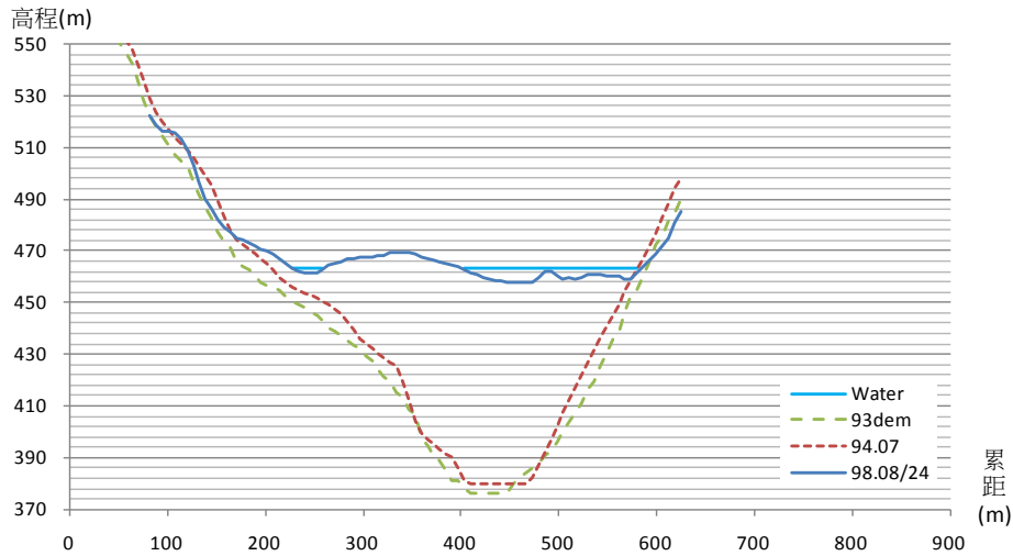
水下地形測量成果斷面 A1
