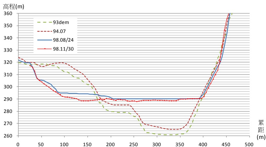
太麻里溪河道斷面比對斷面 14
