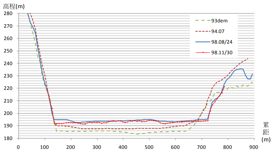
太麻里溪河道斷面比對斷面 12
