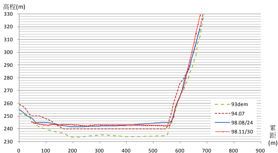
太麻里溪河道斷面比對斷面 13
