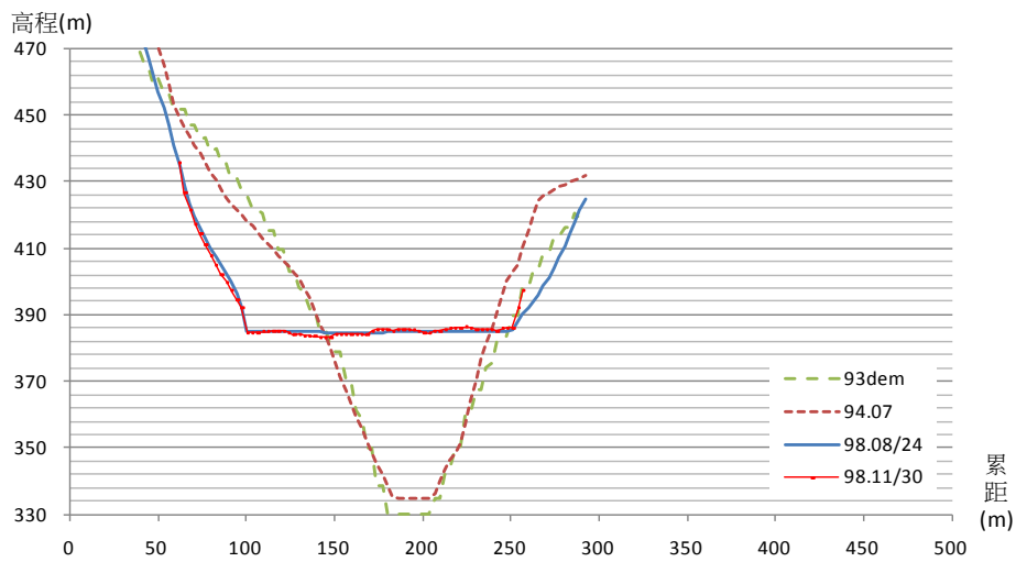
太麻里溪河道斷面比對断面 20
